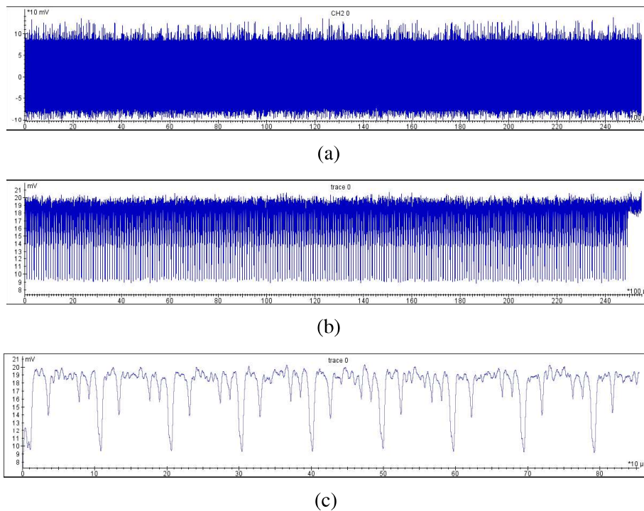
Figura 3.13: Trace de radiação eletromagnética de uma execução de ECSM com algoritmo Montgomery Ladder: (a) original não filtrado; (b) após aplicação de filtro baixa e (c) zoom no início deste último. Traces processados com Inspector [Riscure 2016].
