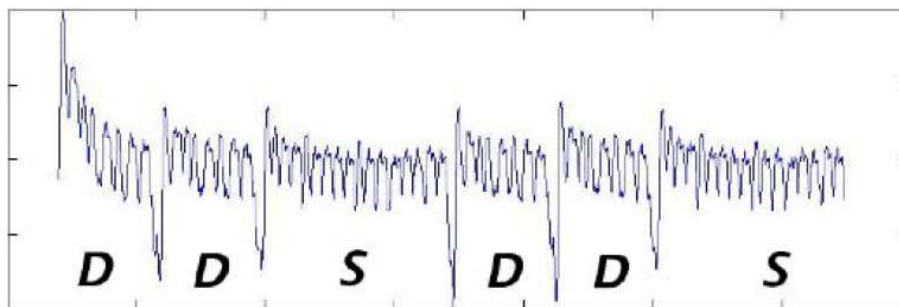
Figura 3.10: Consumo de potência durante cálculo de kP [Hankerson et al. 2004].
