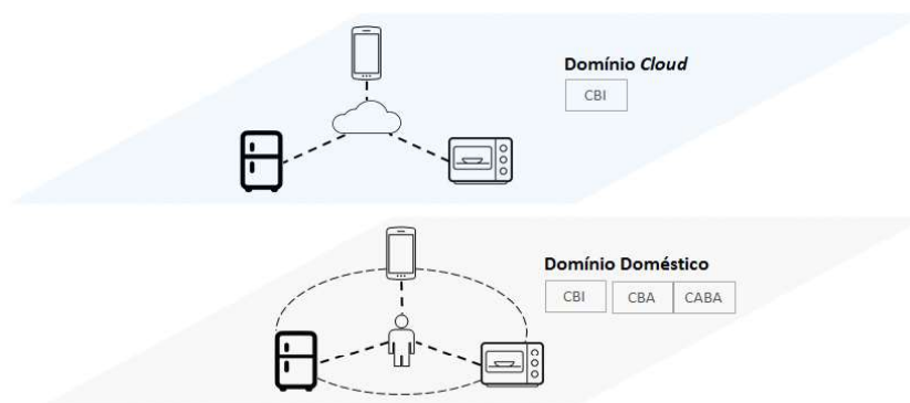
Figura 1. Arquitetura de dois domínios do AdC.
